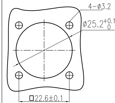
面板开孔图
