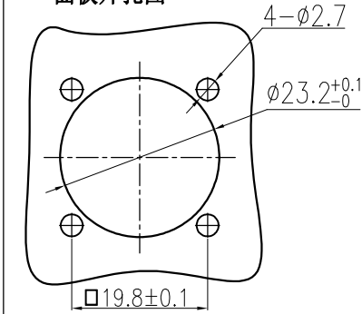
面板开孔图
