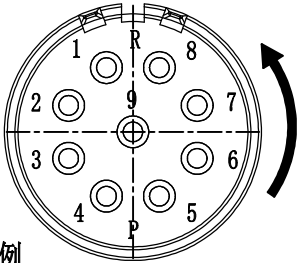
针位排布图
