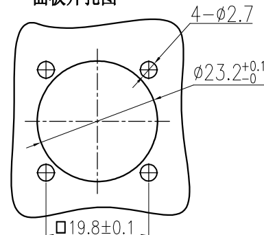
面板开孔图
