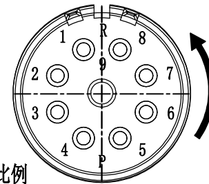
针位排布图
