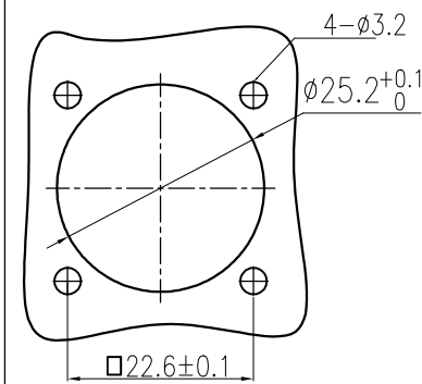
面板开孔图
